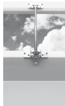
Manueller Öffner, Wanderspindel
